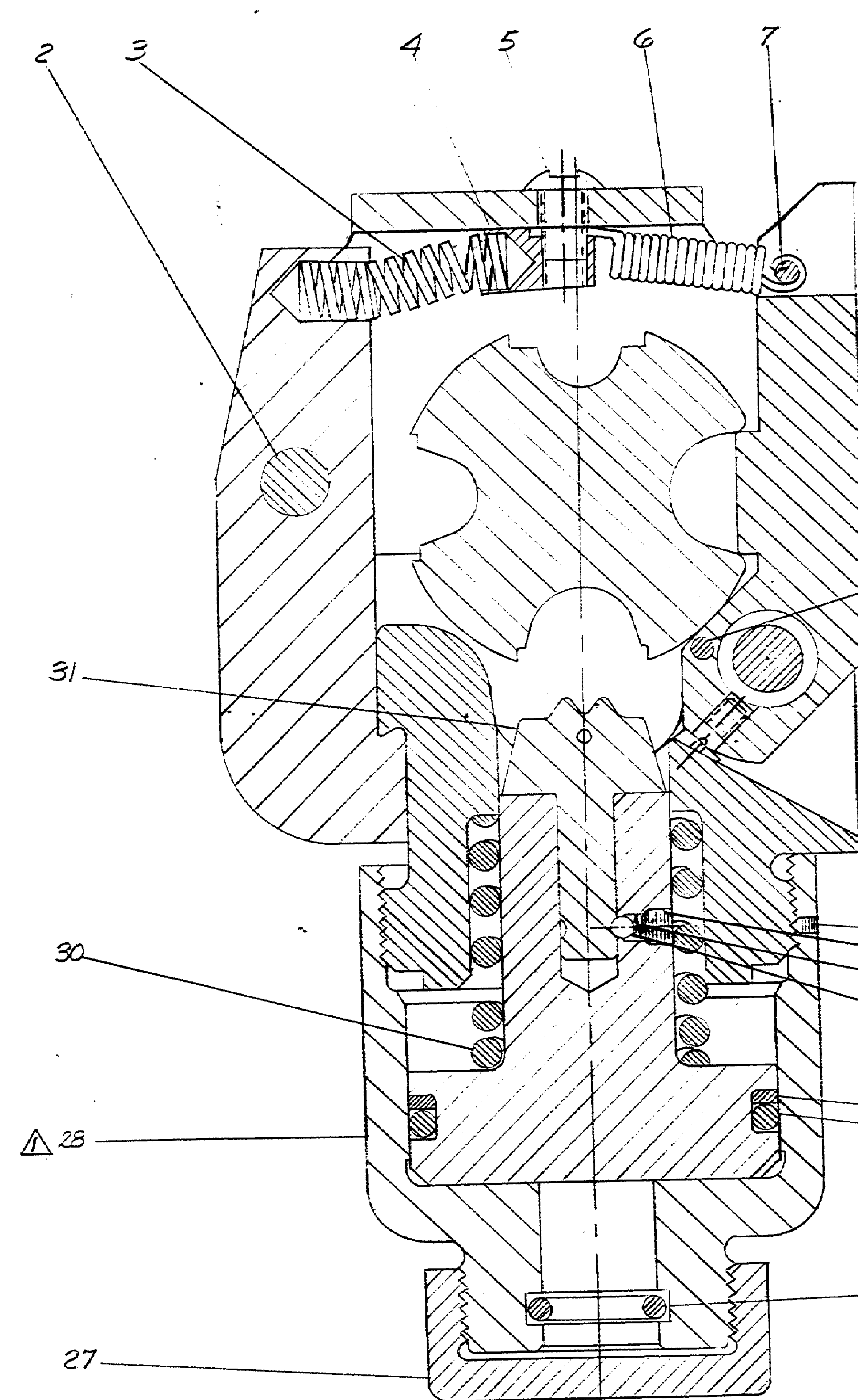
SECTION A-A
