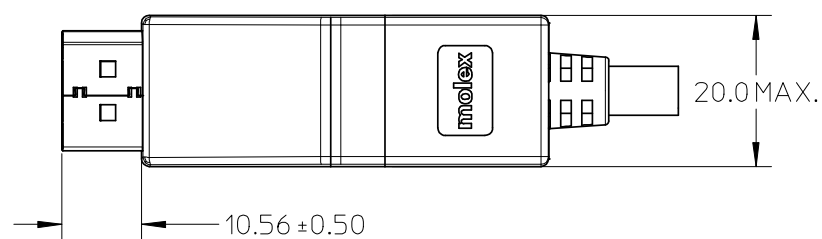
BACK SIDE P1 (DISPLAYPORT M)
