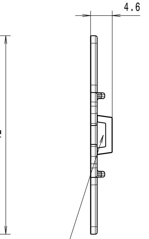
Aufnahme fuer Kabelbinder/ Retainer for cable tie (4.9 x 1.6)
