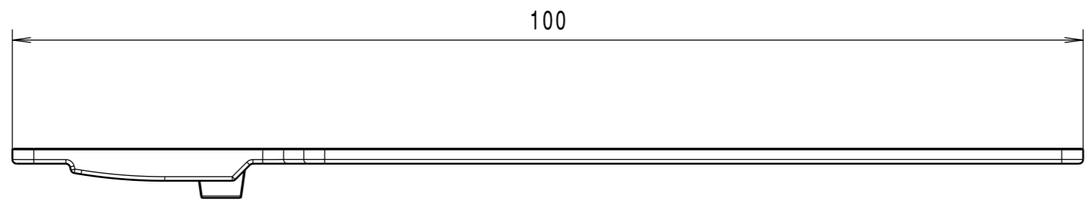
Aufnahme fuer Kabelbinder/ Retainer for cable tie (4.9 x 1.6)
