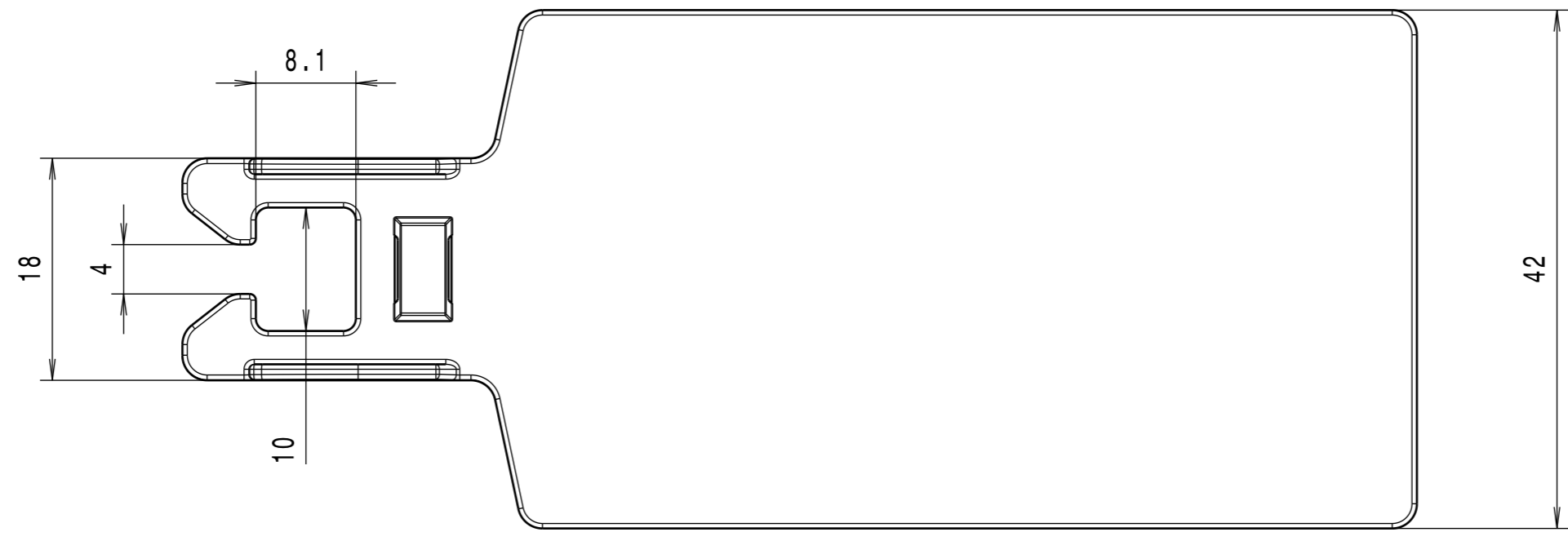
Aufnahme fuer Kabelbinder/ Retainer for cable tie (4.9 x 1.6)
