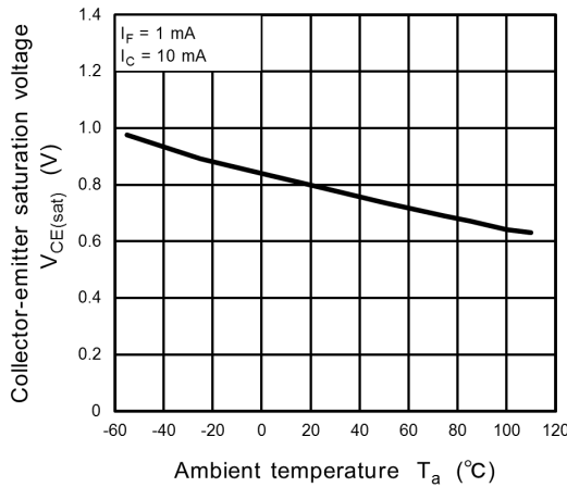
Fig. 11.9 V_{CE(sat)} - T_a
